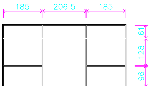
新作鋁合金框架示意圖(4.5*10cm)
